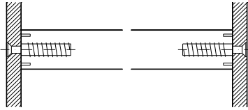
Verbindung Wange-Stufe
