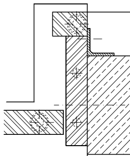
Austrittsbefestigung
