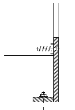
Antrittsbefestigung
