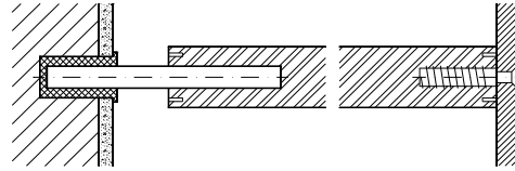
Verbindung Wand-Stufe
